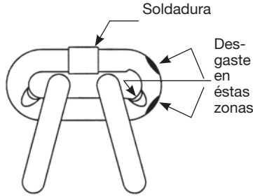
Figura 6 - Inspección de la cadena
