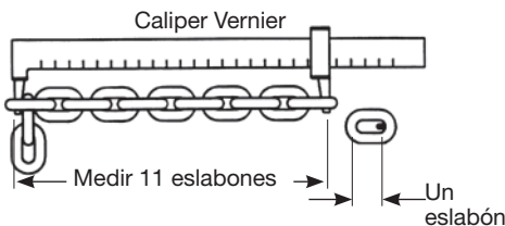
Figura 7 - Inspección de la cadena
