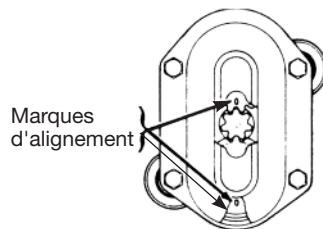
Figure 10 - Alignement d'engrenages
