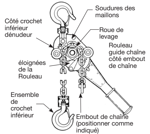
Figure 11 - 3/4, 1, 1½, 2 et 3 tonne
