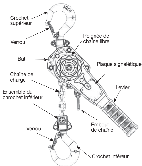
Figure 3 - Parties principales d'un palan à
