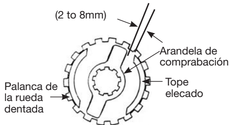
Figura 9 - Posición de la arandela de compravación
