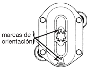
Figura 10 - Orientación de los engranajes
