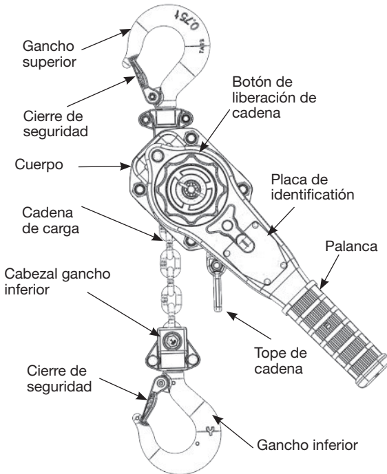
Figura 3 - Partes principales del polipasto de palanca
